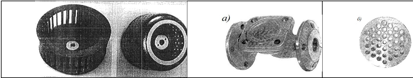
Рис. 1 – Примеры элементов оборудования, гуммированного ЖЭК
