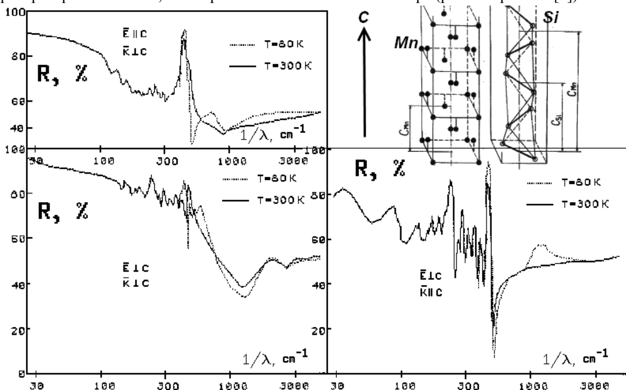
Рис.8. Спектры отражения одномерно-несоразмерного квазикристалла высшего силицида марганца, с двумя несоразмерными кристаллическими подрешётками марганца и кремния и модель его кристаллической решётки.
