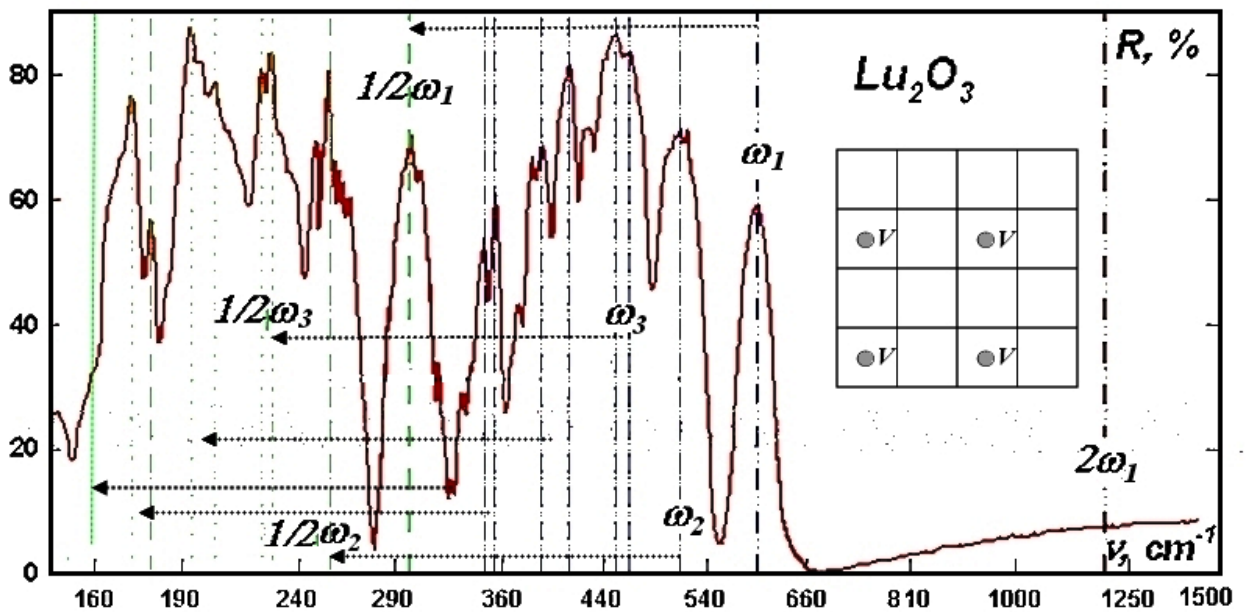
Рис.7. Спектры Решёточного Отражения кристалла окисла лютетия, с ещё более сложной, с регулярно расположенной в элементарной ячейке вакансиями с соразмерным кристаллической ячейке периодом трансляции, тоже описываемой фёдоровской (3х-мерными) группами симметрии (из работы [3]).
