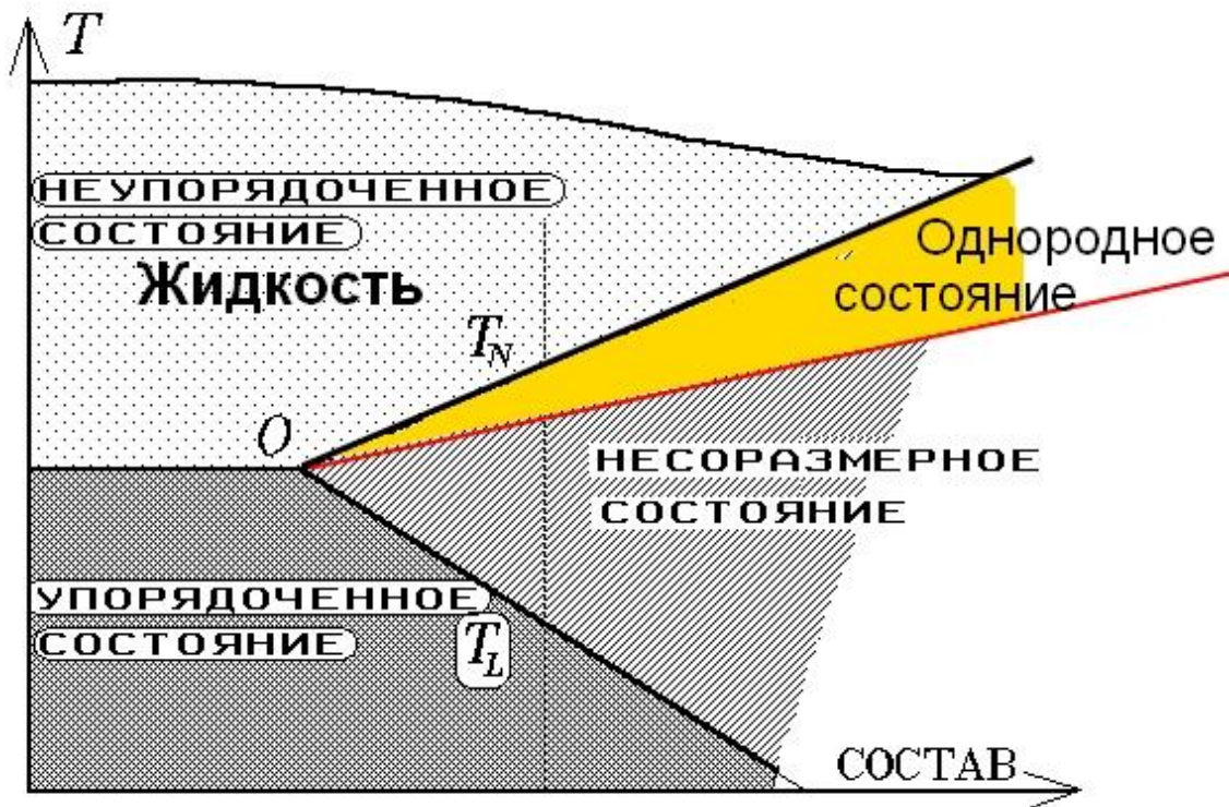
Рис.11. Схема формирования из расплава высоко симметричной однородной фазы, переходящей с понижением температуры в несоразмерную фазу с решёткой концентрационных солитонов.
