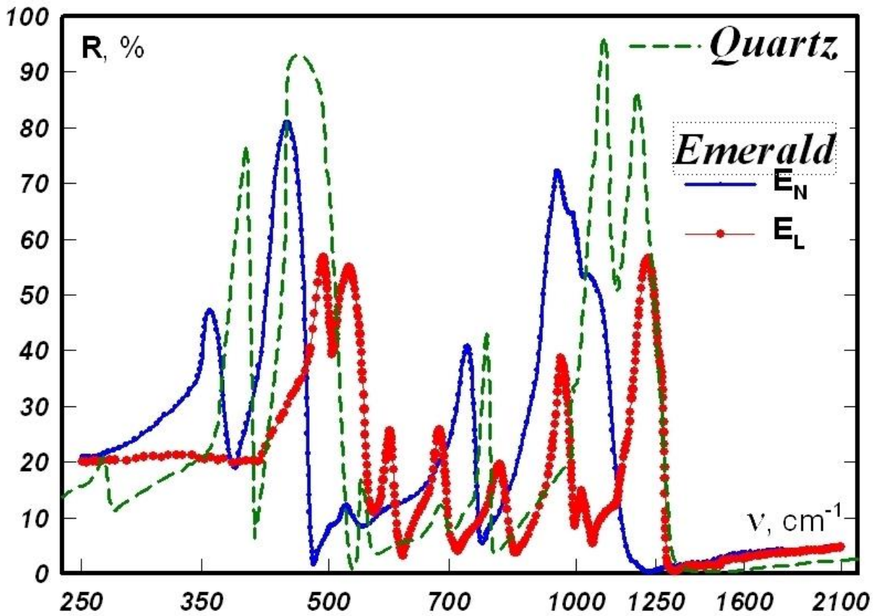
Рис.6. Спектры Решёточного Отражения кристаллов кварца и изумруда, с более сложными кристаллическими решётками, но также соразмерными, описываемыми фёдоровскими (3х-мерными) группами симметрии.
