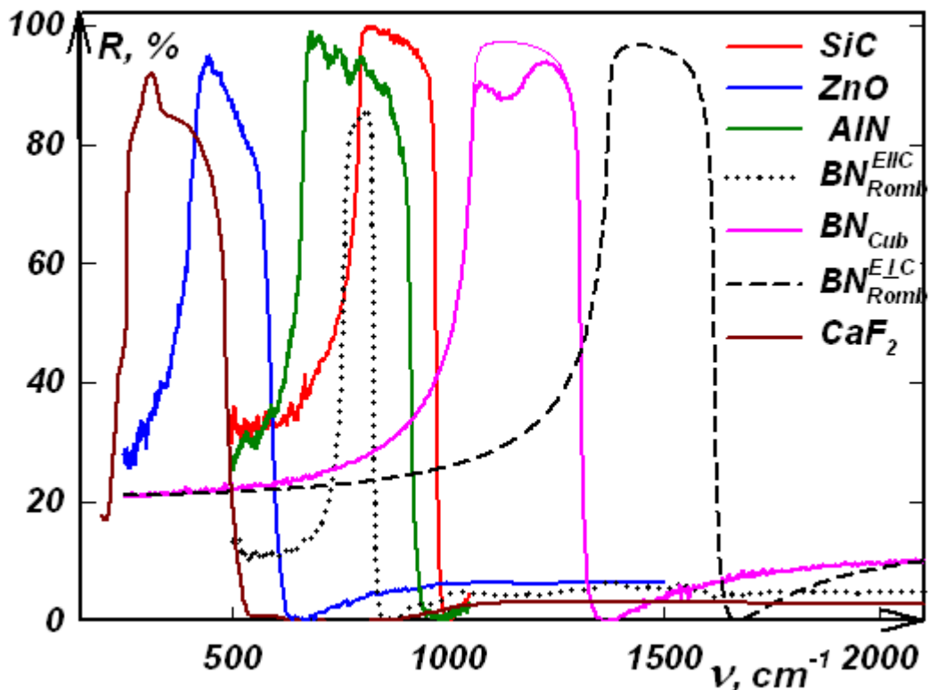
Рис.5. Спектры Решётчного Отражения ряда кристаллов с простейшими (изотропными и с одной осью симметрии у ромбоэдрического BN), с описываемыми фёдоровскими группами симметрии кристаллическими решётками – для BN из работы [2]).
