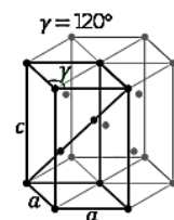
Дважды-объёмноцентрированная (Ромбодрическая)
