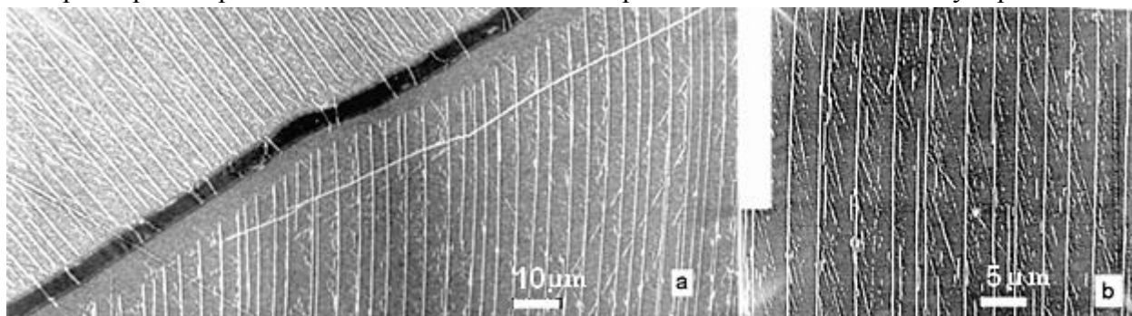
Рис.3. Оптическая фотография в поляризованном свете плоскости параллельной оси С высокоупорядоченных блоков несоразмерных кристаллов высшего силицида марганца, с регулярной решёткой концентрационных солитонов.
